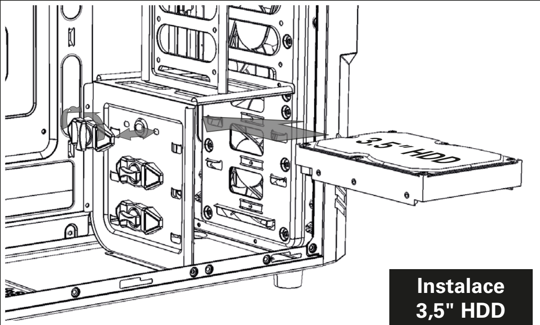
Instalace 3,5" jednotky
